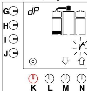
Fig. 17 Programa de primer nivel para la descalcificación del sistema de preparación de café
