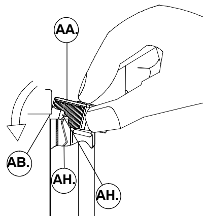
Fig. 9 Colocación y retirada de la tapa del indicador de nivel
